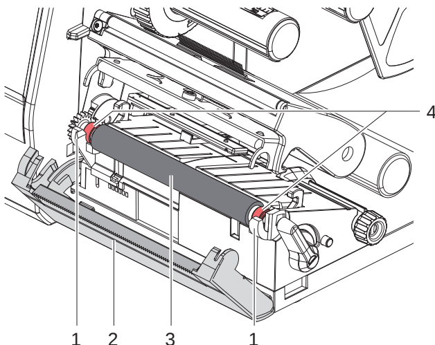
Рис. 15 Печатный валик
