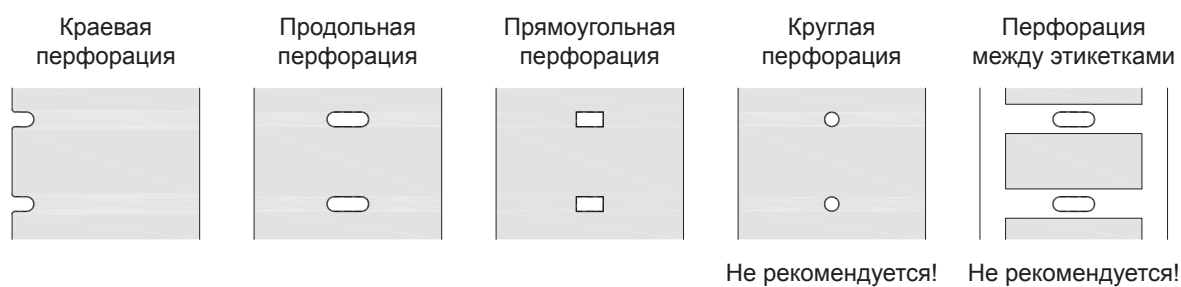
Рис. 22 Примеры перфорации
